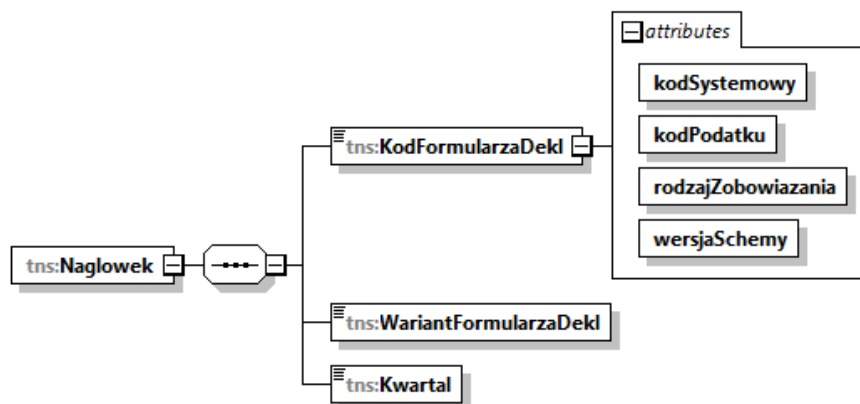
Schemat 15. Struktura Nagłówek w elemencie Deklaracja dla JPK_V7K.
